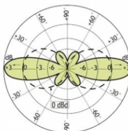
PATRÓN TÍPICO DE RADIACIÓN (PLANO H)
